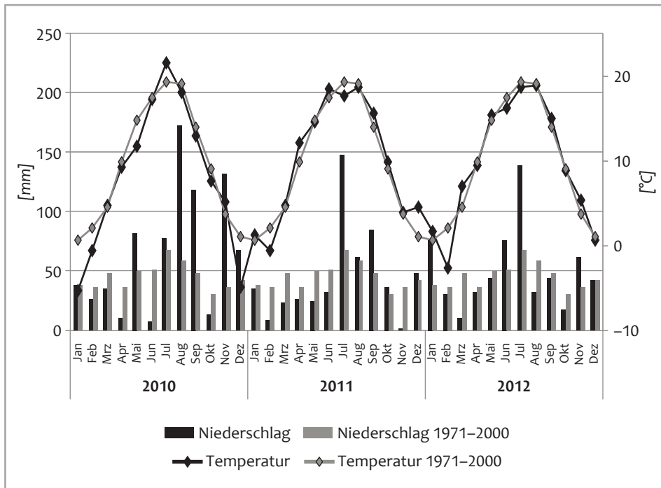
Abbildung 1: Temperaturverlauf und Niederschlagsmengen am Versuchsstandort Pretschen für die Jahre 2010 bis 2012 im Vergleich zum langjährigen Mittel der Referenzperiode 1971 bis 2000 (Klimastation Lübben-Blumenfelde) (Quelle: DWD).
