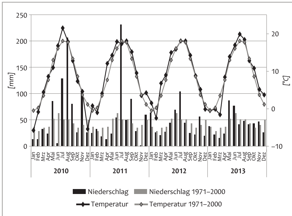
Abbildung 2: Temperaturverlauf und Niederschlagsmengen am Versuchsstandort Münchenber für die Jahre 2010–2013 im Vergleich zum langjährigen Mittel der Referenzperiode 1971–2000 (Klimastation Münchenber; Quelle ZALF)
